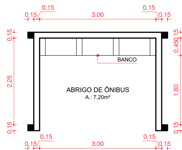
01 PLANTA BAIXA ESC.: 1/50
