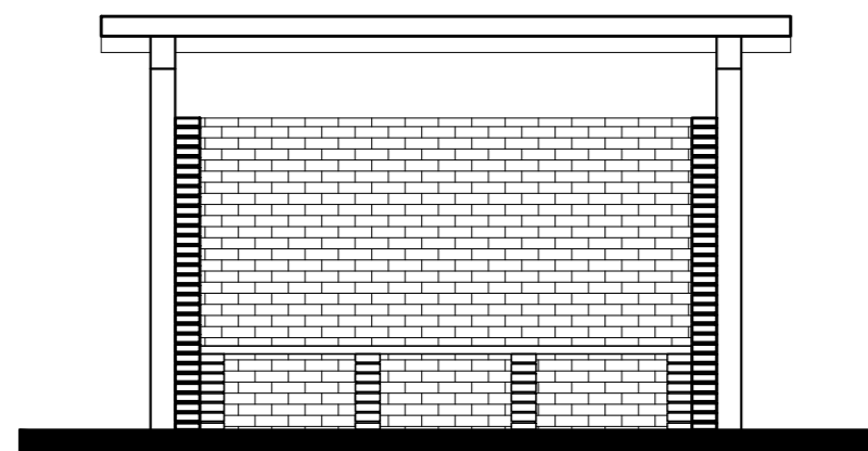
03 FACHADA FRONTAL ESC.: 1/50
